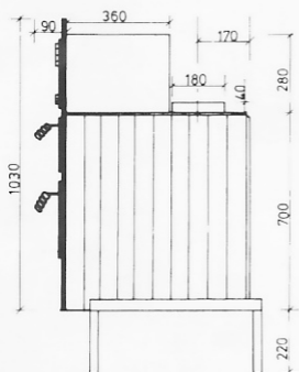
Seitenansicht
